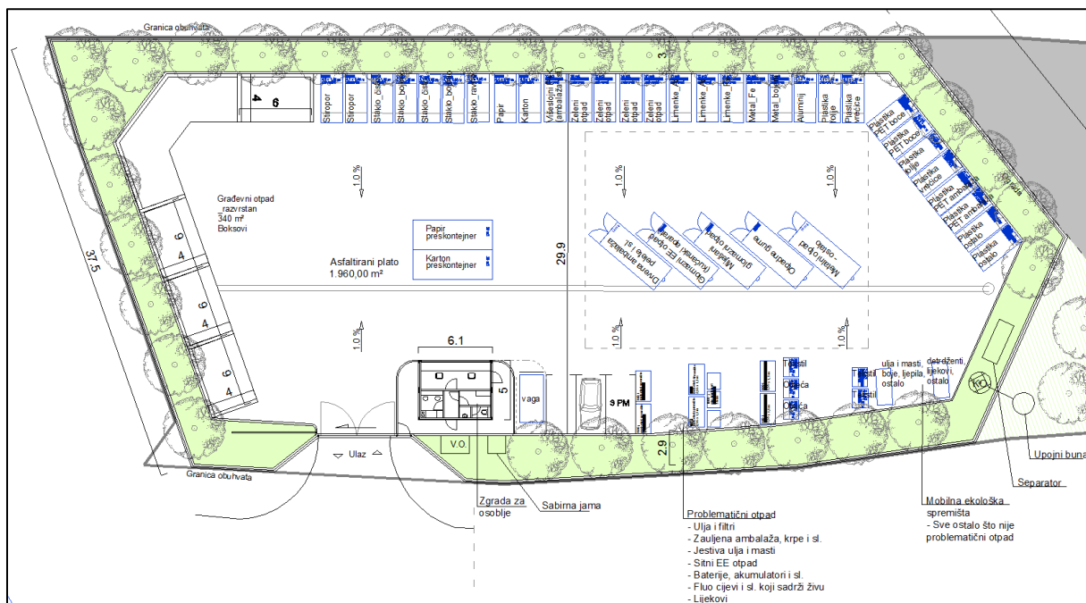
Slika 4: Prikaz reciklažnog dvorišta – varijantno rješenje
